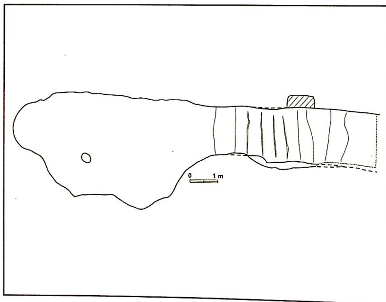
Obr. 3: Půdorys lochu se schodištěm. Šrafovaně je vyznačeno smíšené zdivo dozdivky, čárkovaně zakrytý nebo předpokládaný průběh půdorysu, tečkovaně okraj odkryté plochy. Do půdorysu lochu je promítnuta poloha větracího otvoru.
