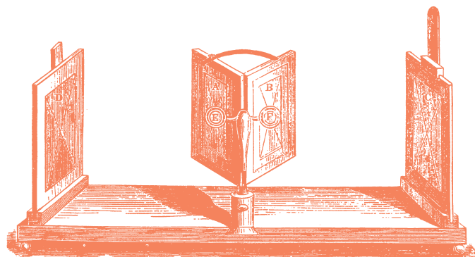
Ukázka zrcadlového stereoskopu (zdroj wikimedia.org/wiki/File:Charles_Wheatstone-mirror_stereoscope_XIXc.jpg )
