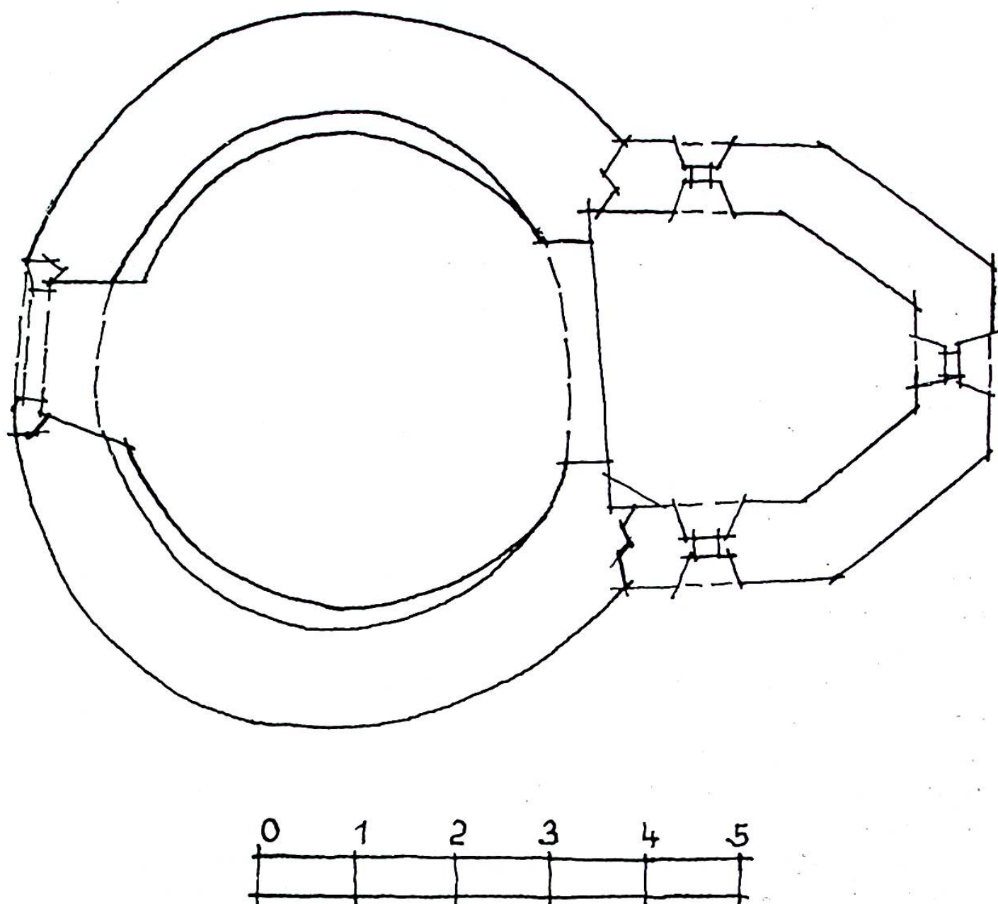
Obr. 3. Karner ve Stonařově. Vyměřil ing. architekt J. Mannsbarth.
