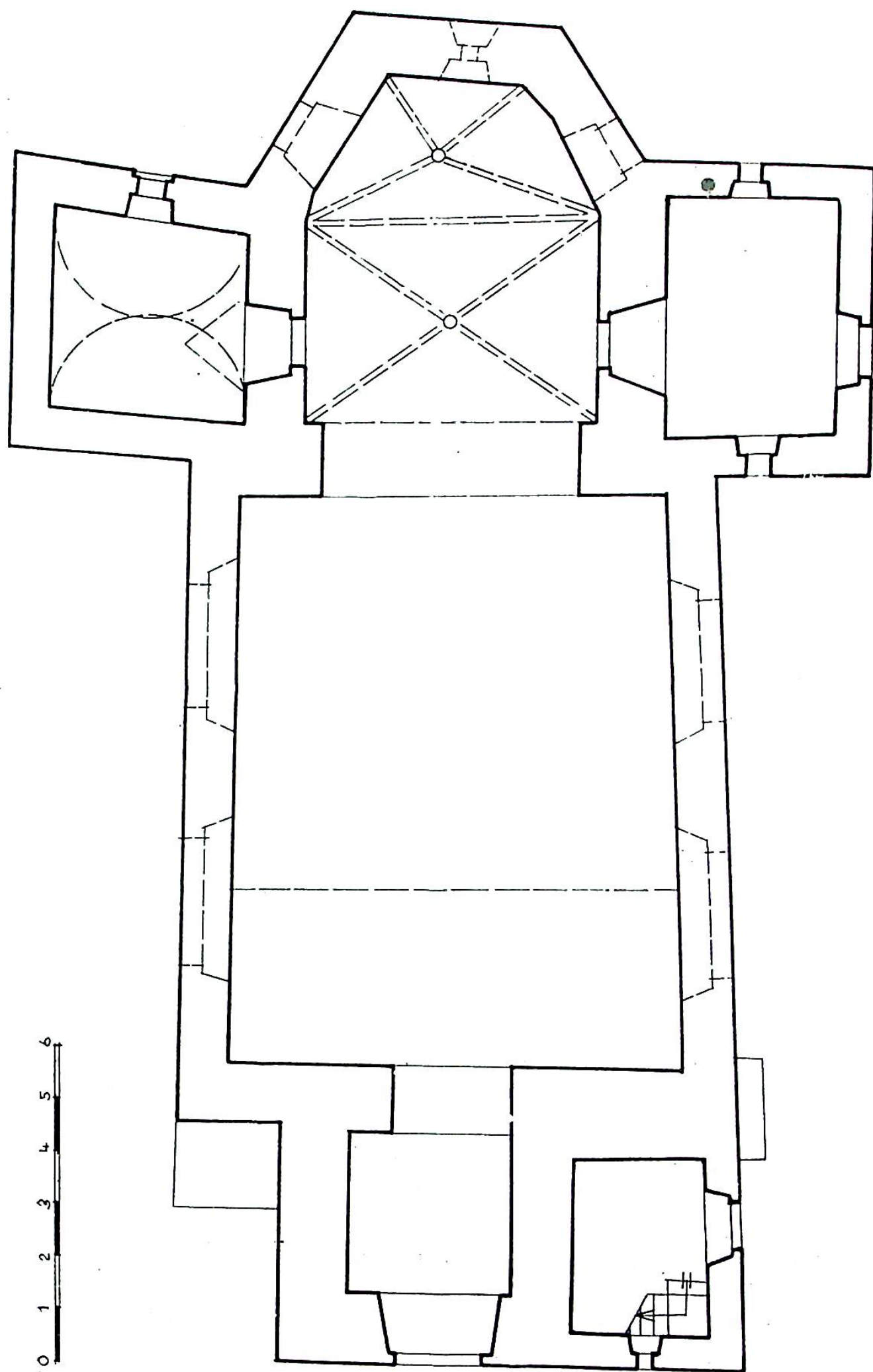
Obr. 4. Farní kostel sv. Jakuba ve Vilánci. Vyměřil ing. architekt J. Mannsbarth.
