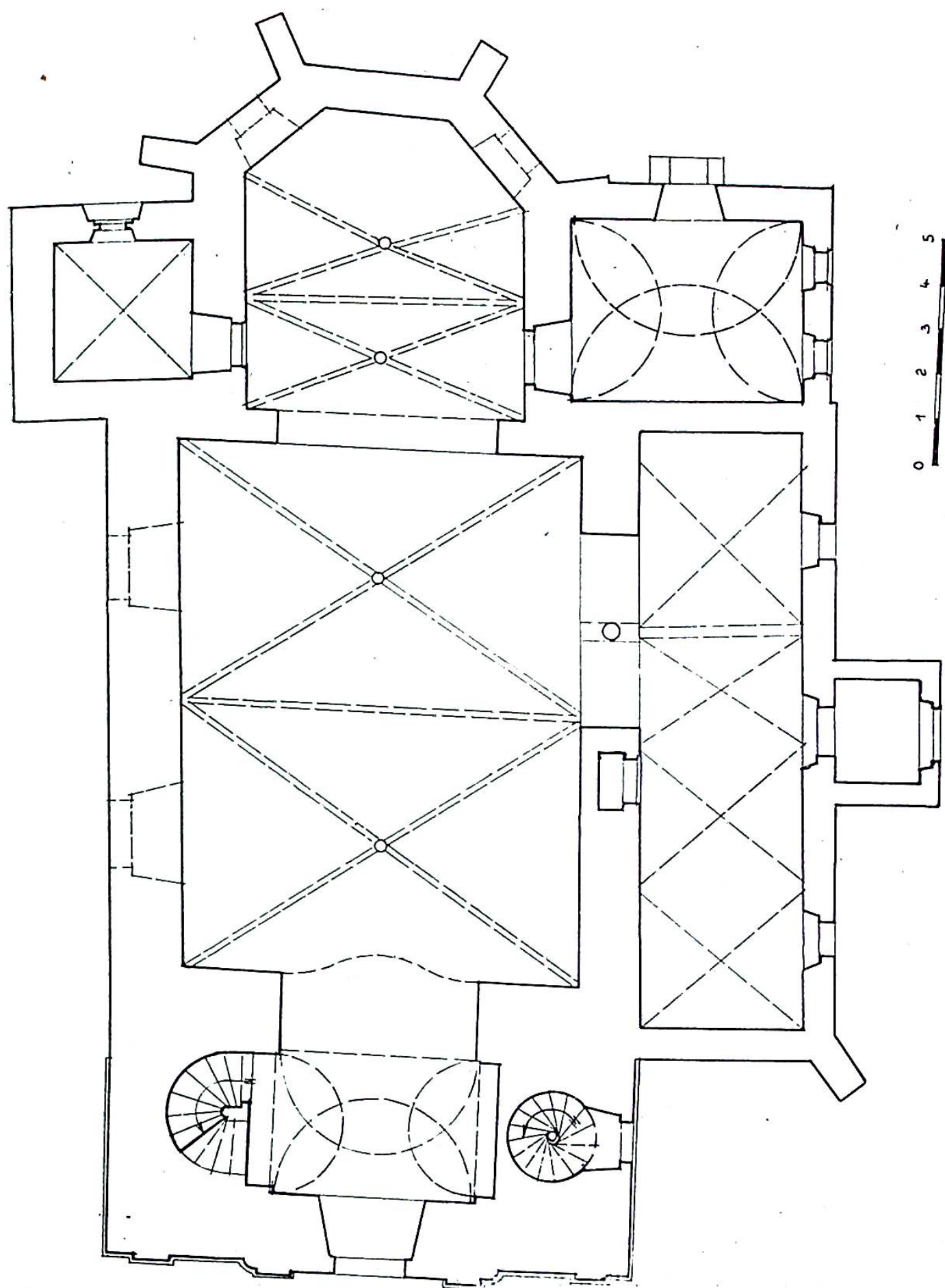
Obr. 1. Farní kostel sv. Petra a Pavla v Rancířově. Vyměřil ing. architekt J. Mannsbarth.
