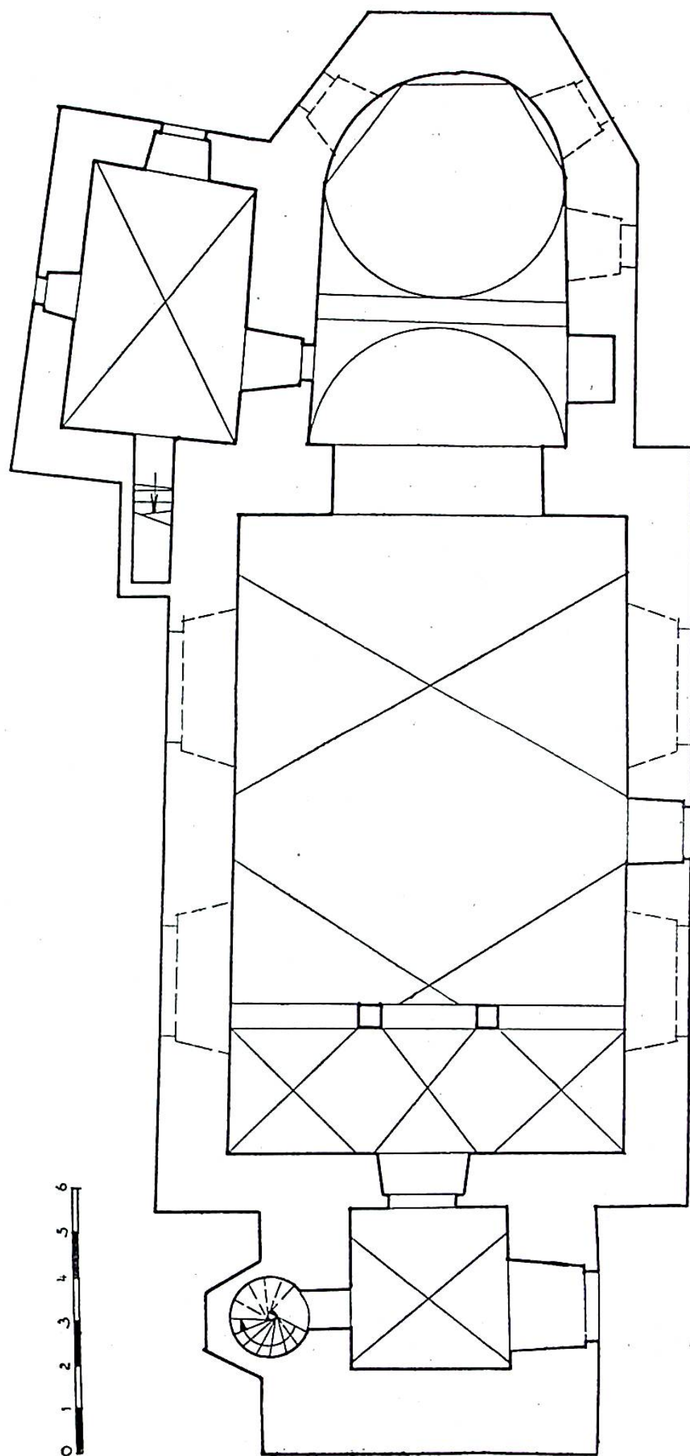
Obr. 2. Farní kostel sv. Václava ve Stonařově. Vyměřil ing. architekt J. Mannsbarth.
