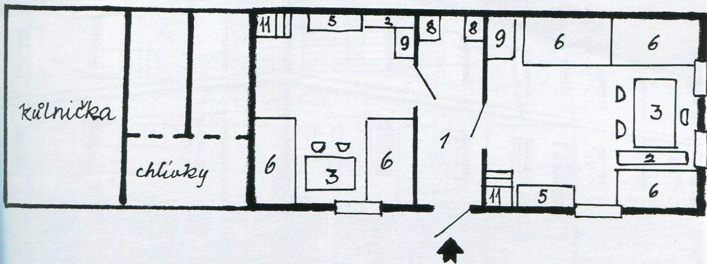
5. Chudobinec ve Velkém Rybníku (v levé i pravé části žil stejný počet lidí, vždy 2 dospělí a 3 děti), stav ve 30. letech 20. století; nejčastější půdorys a členění chudobinců. Měřítko 1 : 100. Legenda: 1 – chodba, 2 – lavice, 3 – stůl a židle, 5 – kredenc, 6 – postel, 8 – stravní almárka, 9 – truhla, 11 – kamna .
