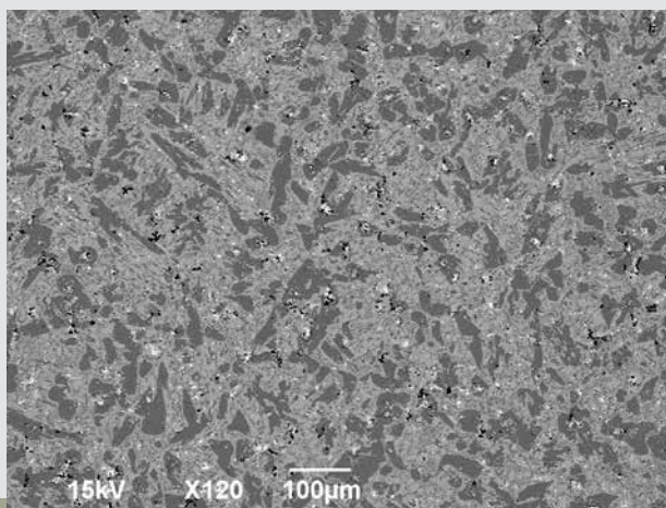
Struktura zvonoviny v elektronovém mikroskopu
